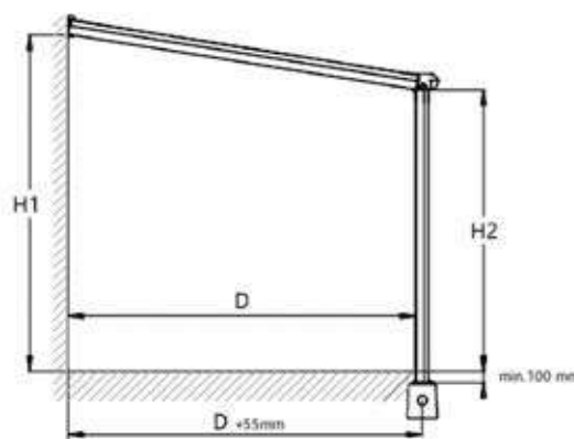
Tekening zijkant
