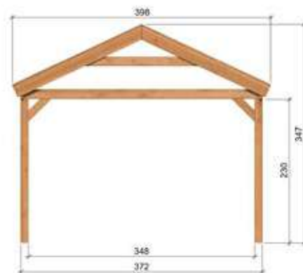
Zijaanzicht
