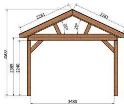
Zijaanzicht XL
