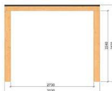
Zijaanzicht
