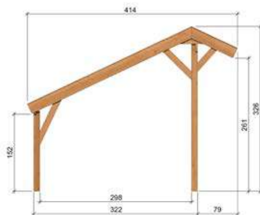
Zijaanzicht
