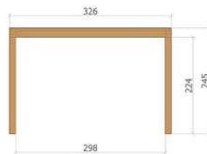
Zijaanzicht L
