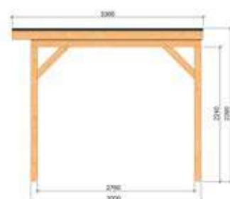
Zijaanzicht
