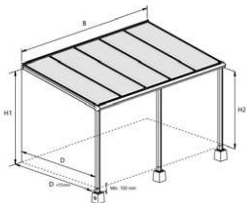
Tekening 3D
